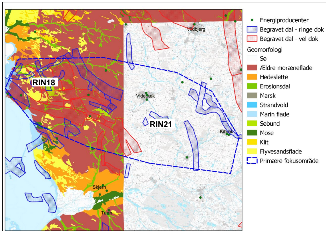
Figur 2.5. Geomorfologisk kort over det undersøgte område. Området er beliggende på en ældre moræneflade. På kortet er ligeledes vist begravede dale (rød og blå skravering) og energiproducenter (grønne punkter, tema fra Dansk Fjernvarme, 2019).
