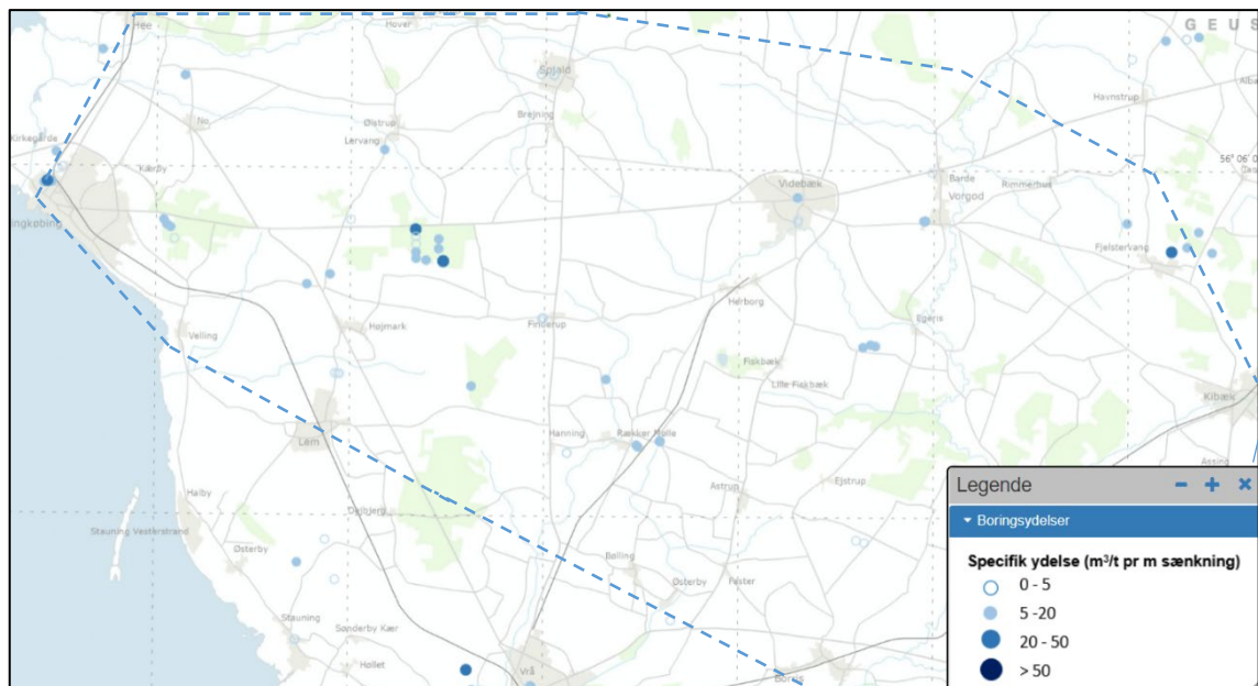
Figur 3.5. Specifikke filtertydelser fra boringer dybere end 100 m i området (m 3 vand/t pr m sænkning) (GEUS varme-lagring). Den blå, stiplede linje angiver fokusområdet.
