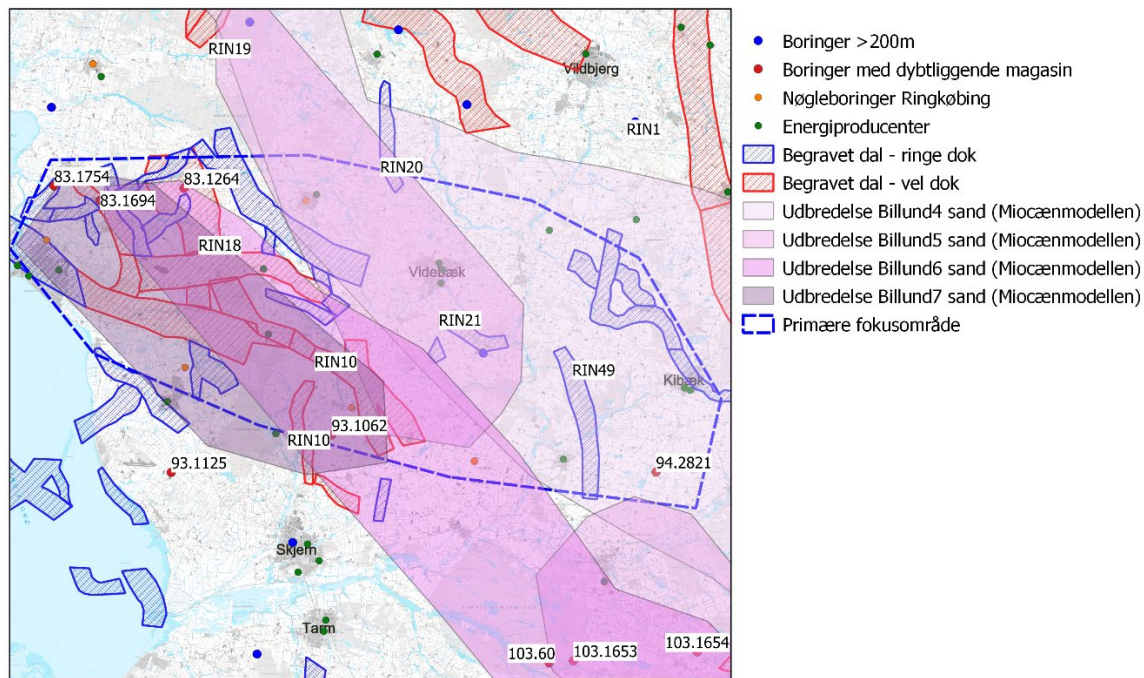
Figur 3.4. Boringer fra Jupiterdatabasen, der anorer dybtliggende sandmagasin (markeret med rødt og DGU nr.). Maksimale udbredelse for tilstedeværelsen af dybtliggende magasin, som er tolket overordnet i Miocæn-modellen (Kristensen et al., 2015) er vist som polygoner.
