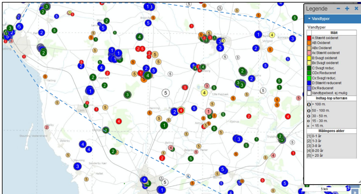
Figur 3.6. Oversigt over beregnede vandtyper, der indirekte fortæller om grundvandskemi og grundvandsmagasinets kontakt til overfladen ( GEUS varmelagrings ). Den blå, stiplede linje angiver fokusområdet.
