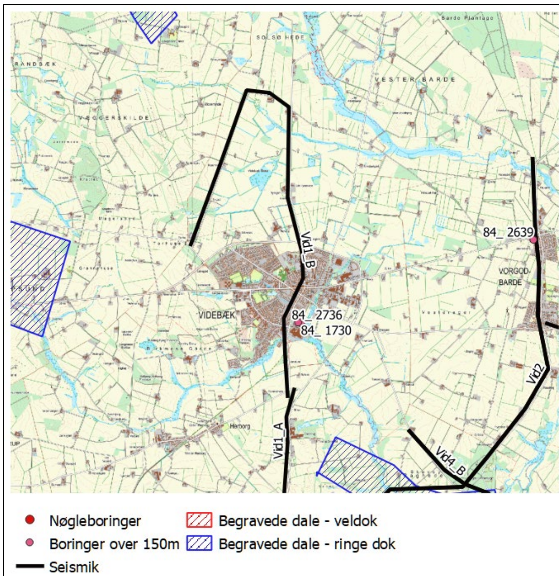
Figur 3.9. Placering af begravede dale, seismiske profiler og dybe borer omkring Videbæk.
