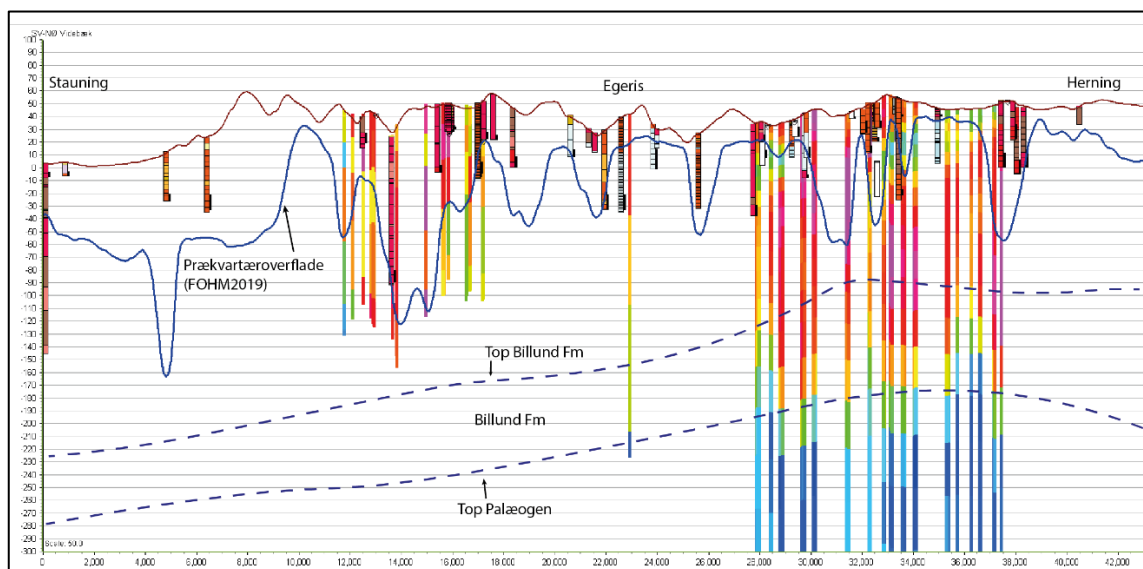
Figur 3.3. Sydvest-nordøst profil fra Stauning over Egeris til Herning med skitsering af den tolkede prækvartære overflade (Miljøstyrelsen, FOHM, 2019) og overordnet tolkning af Billund Formationen fra Miocæn-modellen (Kristensen et al., 2015). Borningsdata er fra Jupiter databasen (GEUS, 2020b). SkyTEM data er fra GERDA databasen (GEUS, 2020a) og blålige farver er lave modstande og indikerer lerede aflejringer, mens røde farver er højere modstande og indikerer mere sandede aflejringer. SkyTEM data har generelt svært ved at opløse de miocæne aflejringer, og skal derfor tolkes forsigtigt her. Overhøjning 50x.
